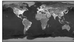
Рис. 5. Ночная Земля
